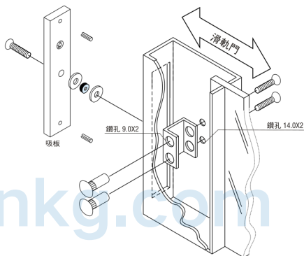
固定螺丝
