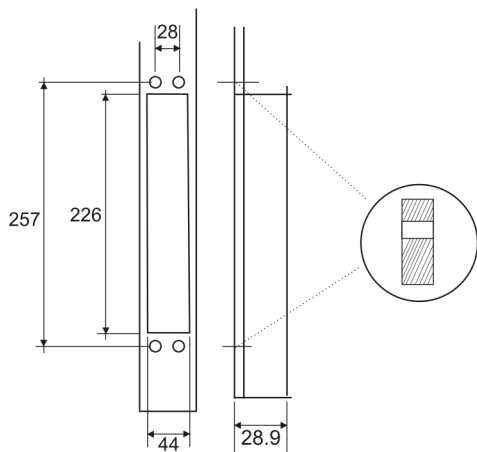
挖空尺寸
