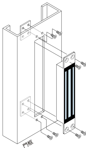
固定螺丝
