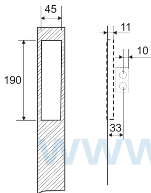
挖空尺寸
